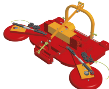
GLM-T
