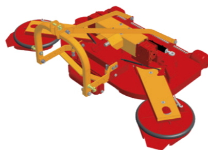
GLM-F
