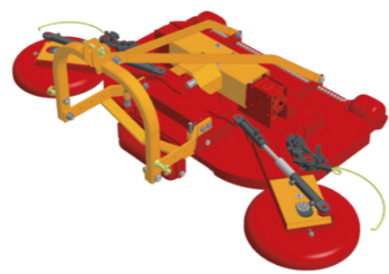
GLM-FT
