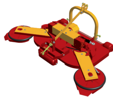
GLM
